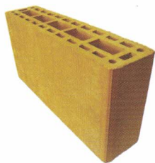
BLOCO ESTRUTURAL 09X19X39
