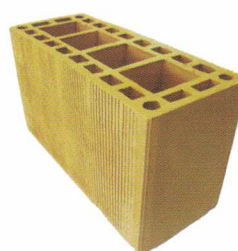
BLOCO ESTRUTURAL 14X19X34
