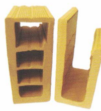
BLOCO CANALETA 11,5X19X31X19 J
