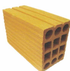
TIJOLO VEDAÇÃO 14X19X29
