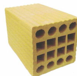
TIJOLO VEDAÇÃO 19X19X29
