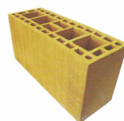
BLOCO ESTRUTURAL 14X19X39
