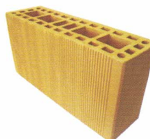
BLOCO ESTRUTURAL 11,5X19X39
