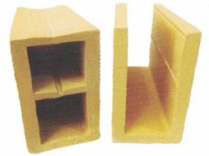
BLOCO CANALETA 11,5X19X29
