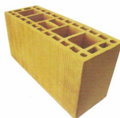
BLOCO ESTRUTURAL 14X12X39
